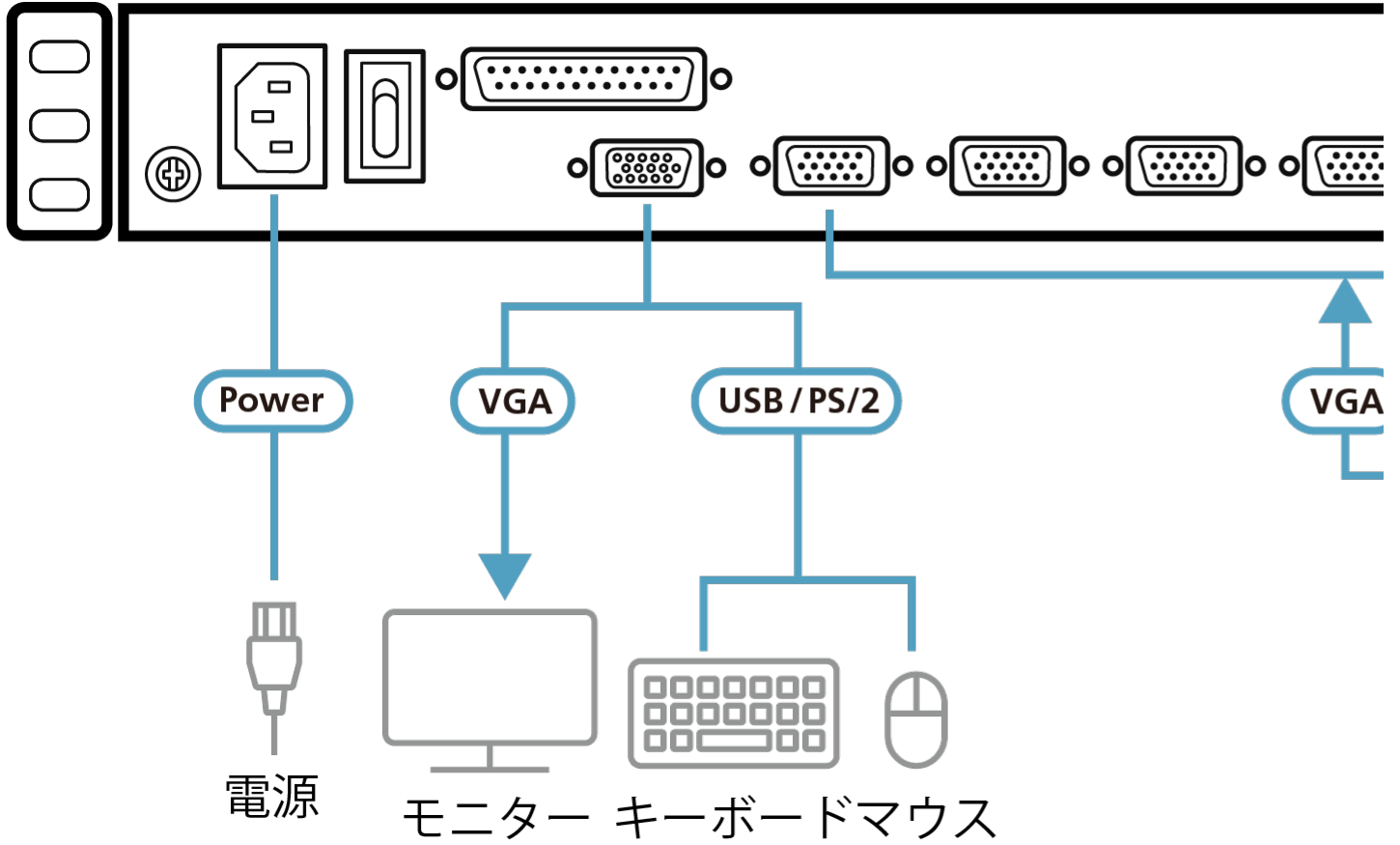
構成図
